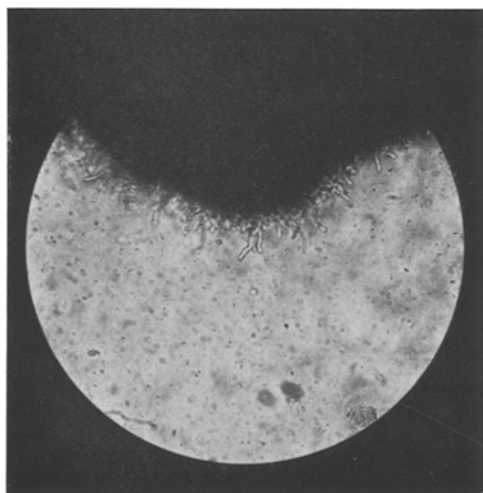
FIG. 2. Normaal kiemend sclerotium op voedingsbodem zonder extract. Germinating sclerotium on nutrition agar without extract.
